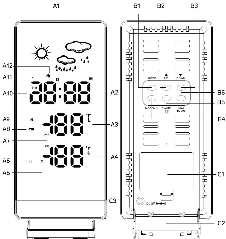
Рис. 1 Схема элементов управления и индикации устройства
